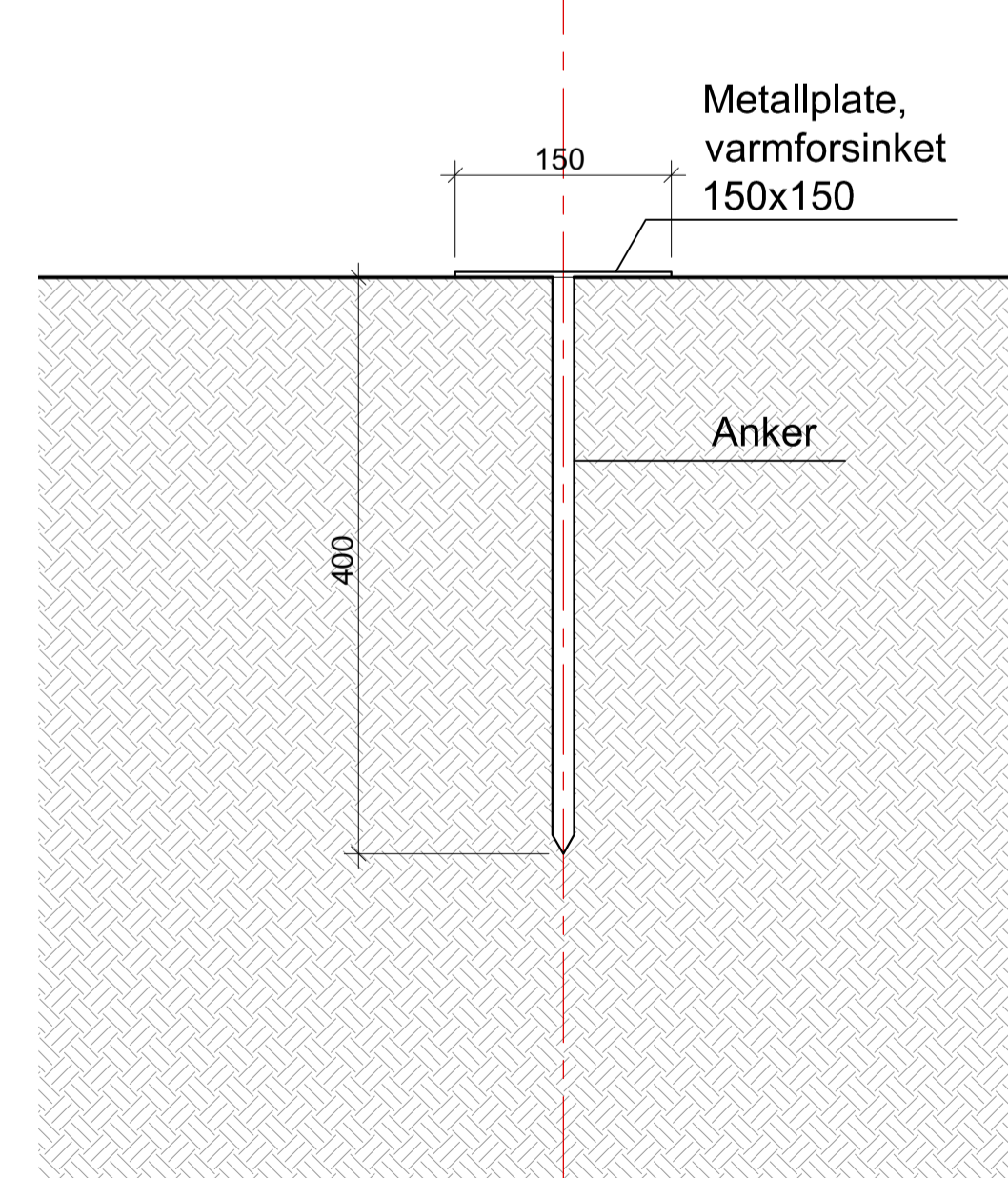
SNITT, METALLPLATE PÅ PARKERINGSPLASS 1:5
