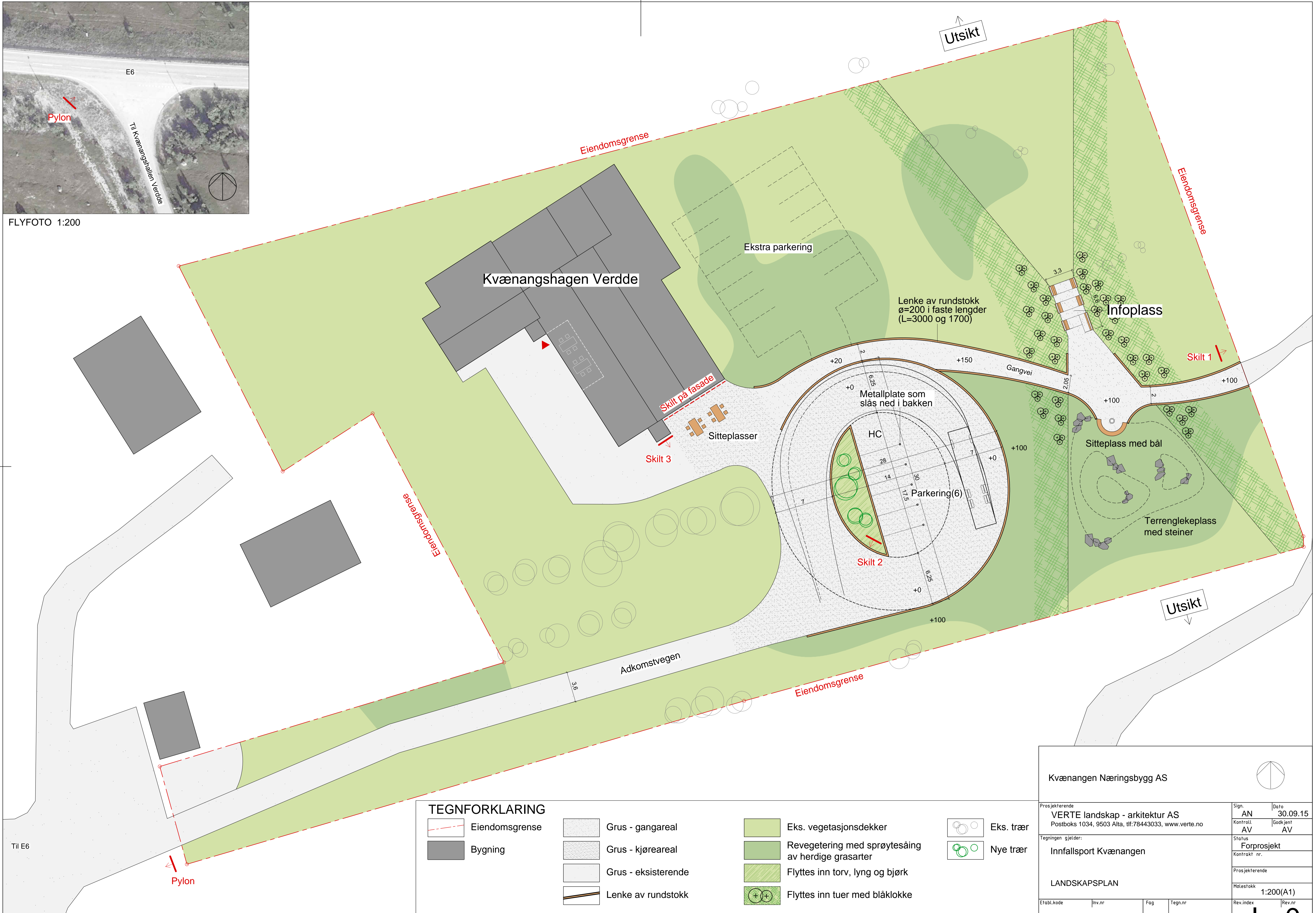
SITUASJONSPLAN 1:200
