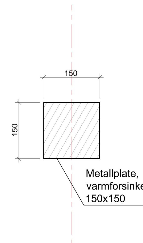
PLAN, METALLPLATE PÅ PARKERINGSPLASS 1:5
