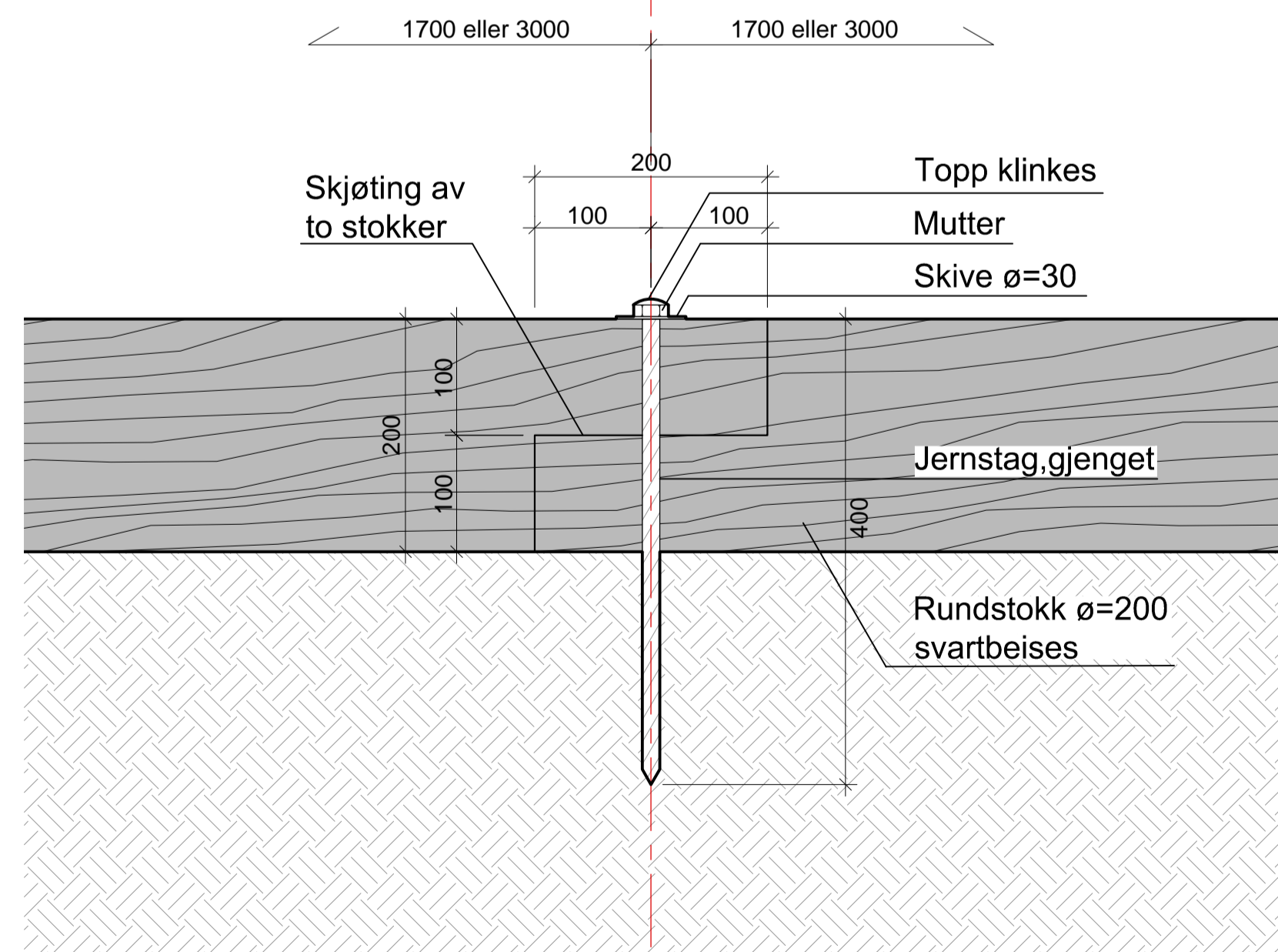
SNITT, RUNDSTOKK 1:5
