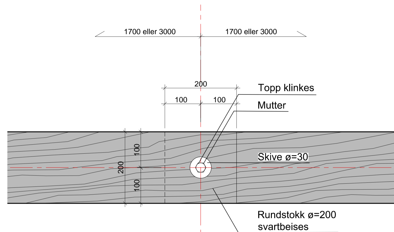
PLAN, RUNDSTOKK 1:5
