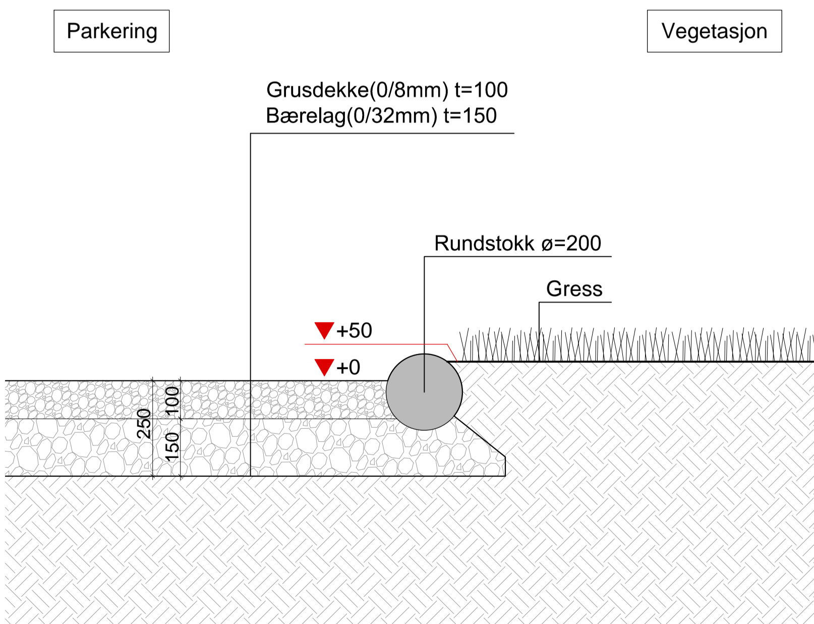
SNITT, KANTTRE PÅ PARKERING 1:10
