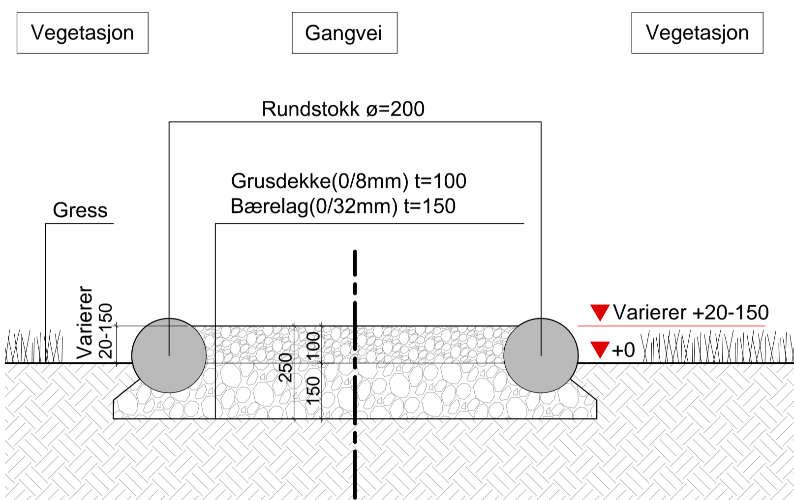
SNITT, KANTTRE PÅ GANGVEI 1:10
