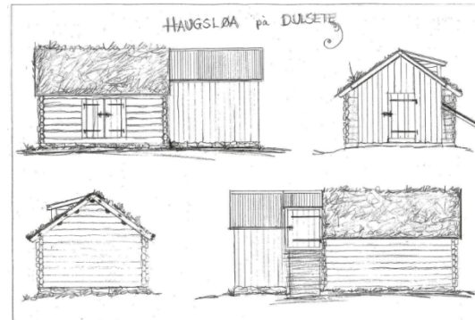
Figur 4 Teikningar av ny "Haugsløa"
