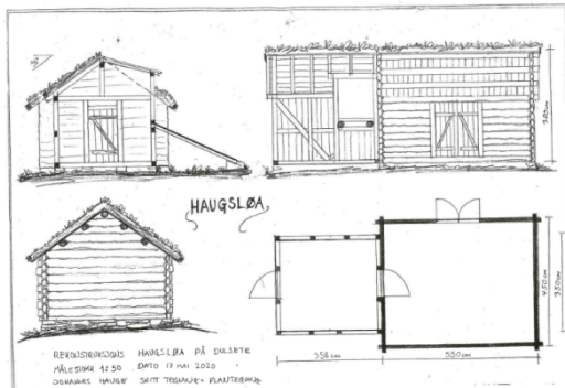
Figur 3 Teikningar av ny Haugsløa på Dulsete.
