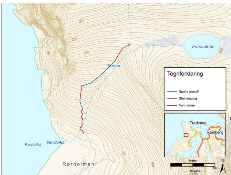
Figur 1. Oversikt over stitrasé og materialvalg.
