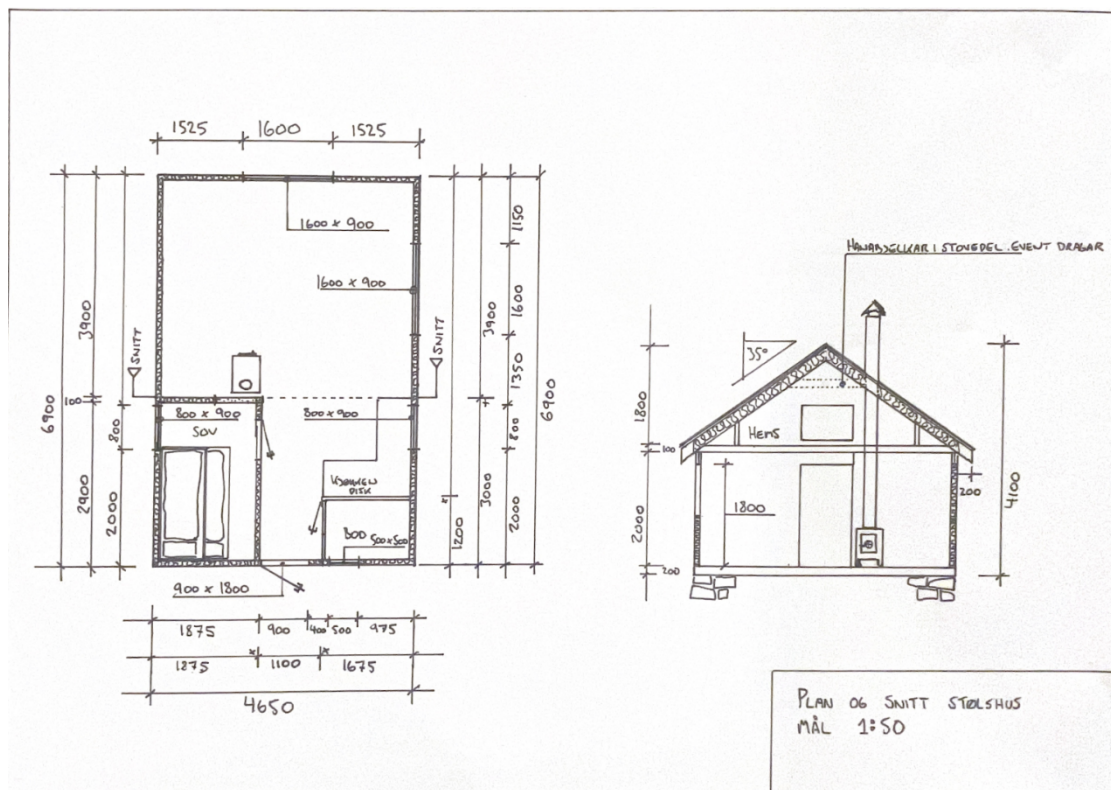
Figur 2 Plan og snitt, stølshus. Kopi frå søknad.
