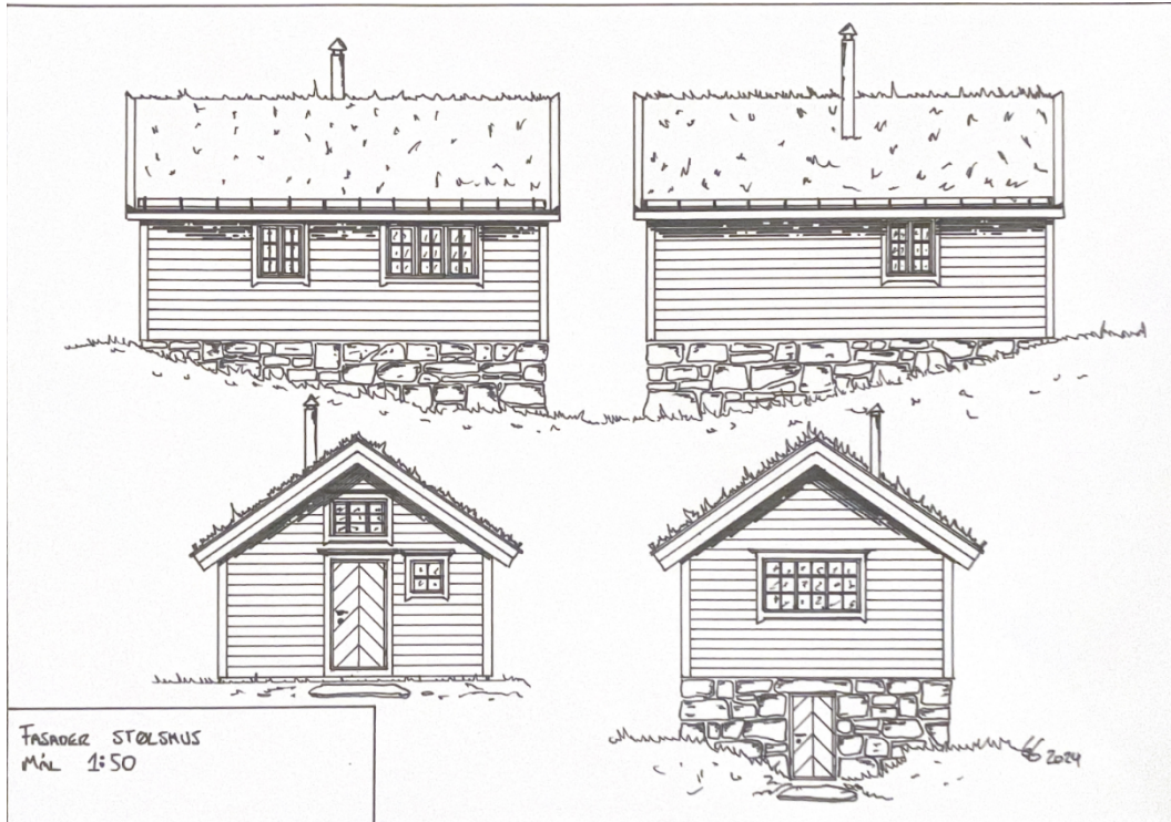
Figur 1 Fasade, stølshus. Kopi frå søknad.
