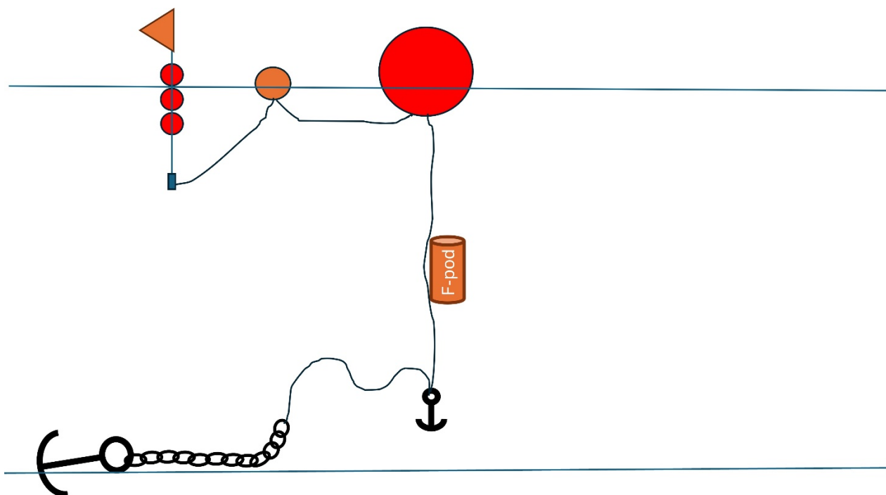
Bilde 2. Skjematisk bilde av forøyning av lydloggere.
