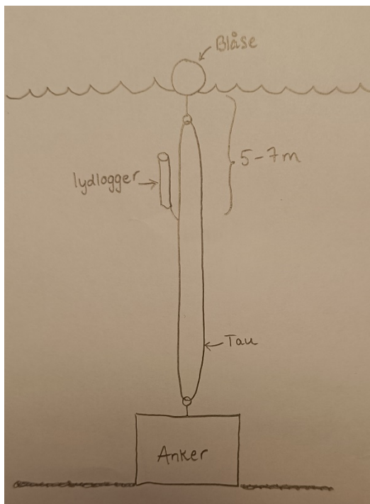
Bild 1. Fortøyning av lydloggere
