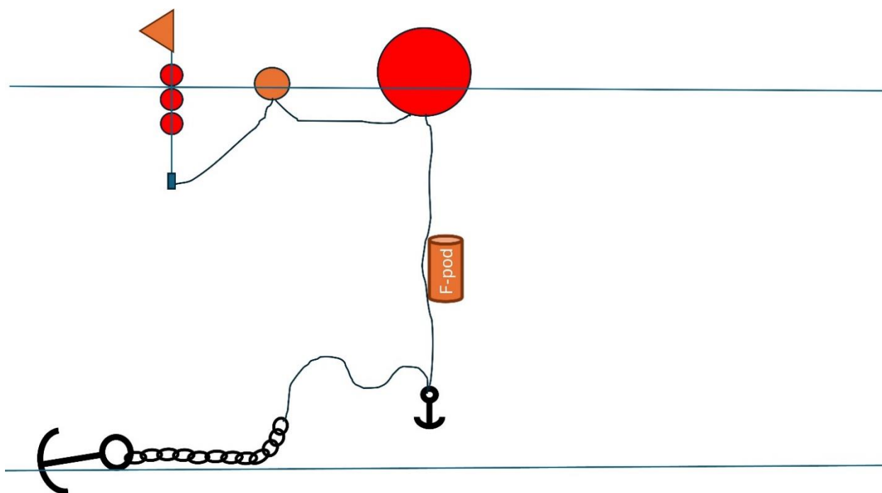
Bilde 1. Fortøying av lydloggeren.
