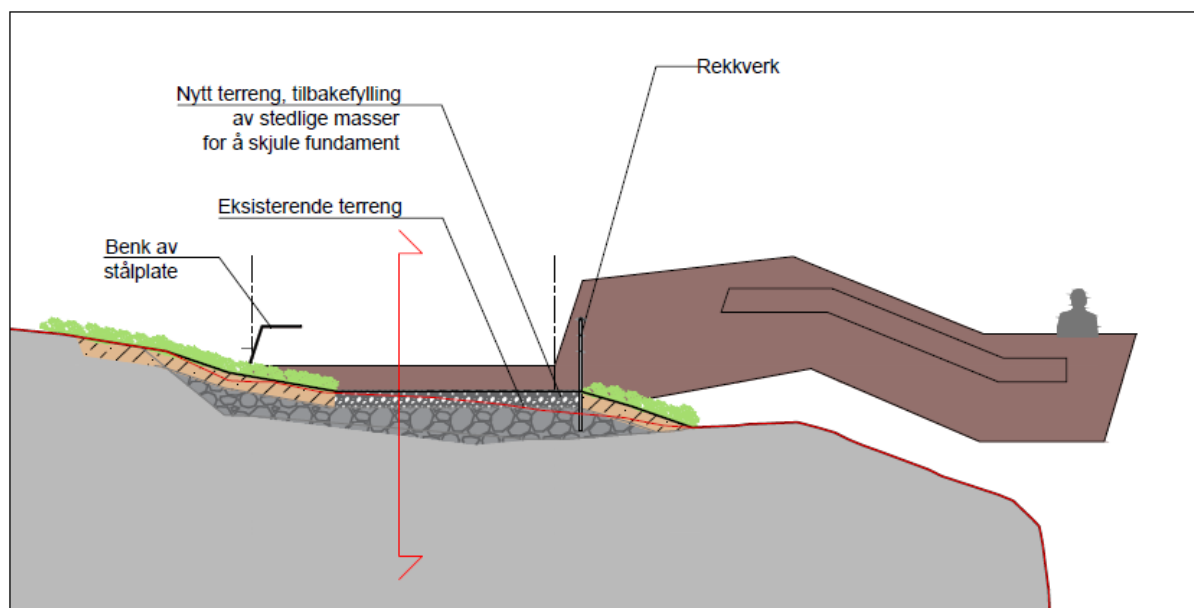
OPPRISS NORDSIDE 1:100
